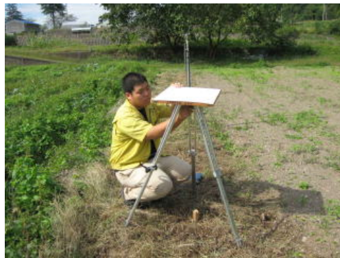
②そこに平板を据え付けます。
